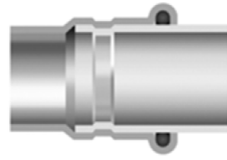
Przekrój połączenia po zaprasowaniu
